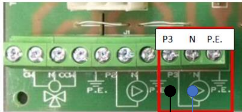
Terminal elektryczny z tyłu kotła.
